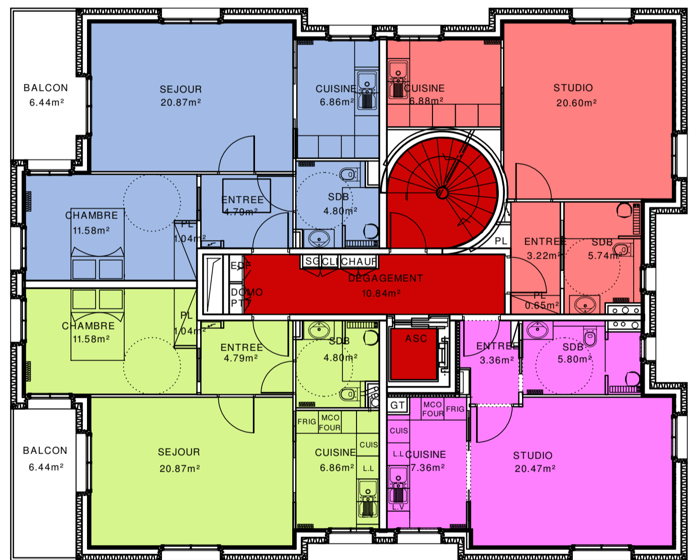
1ER ETAGE
