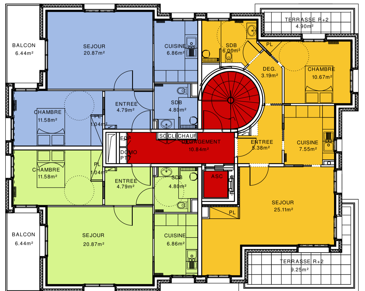
2EME ETAGE
